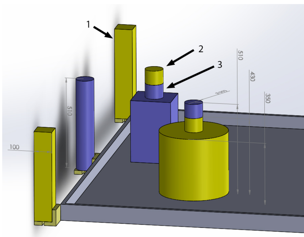
Figure 9 - Exemple de positionnement des balises sur les robots
