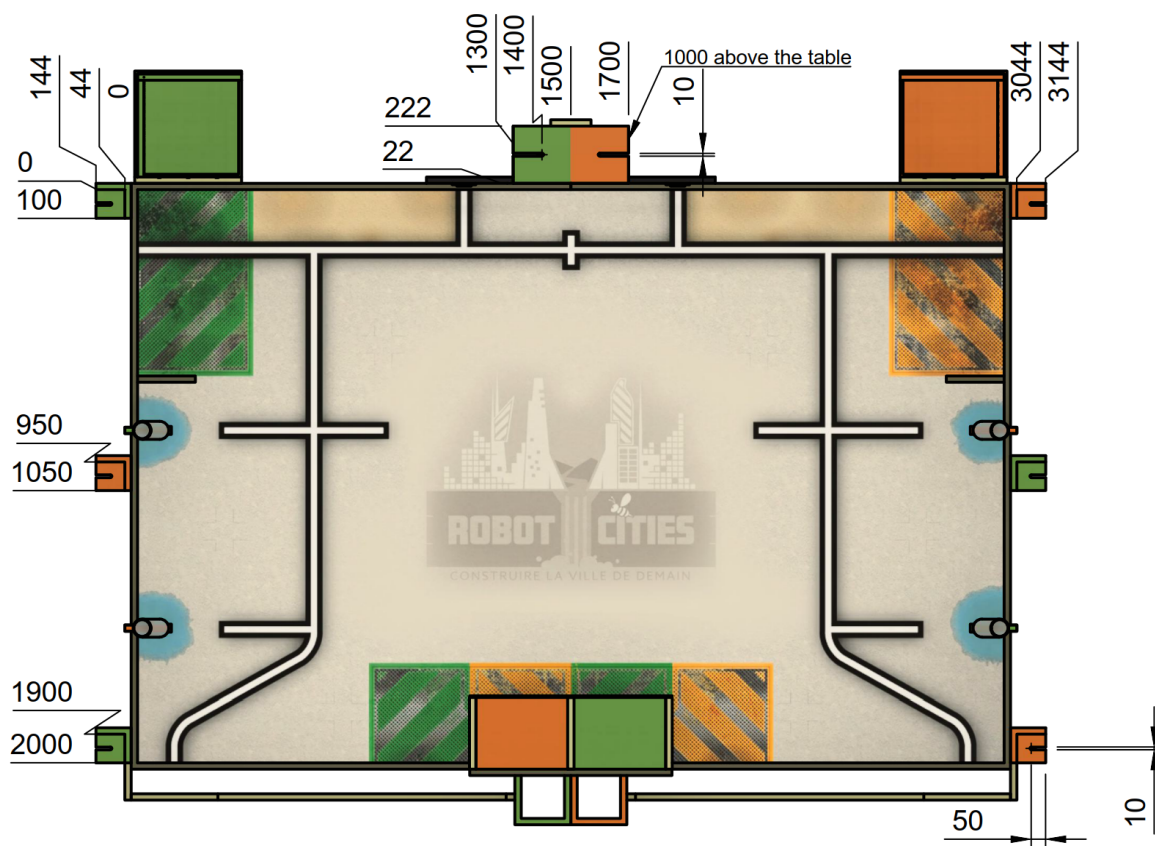
Figure 10 - Positions des balises sur l'aire de jeu
